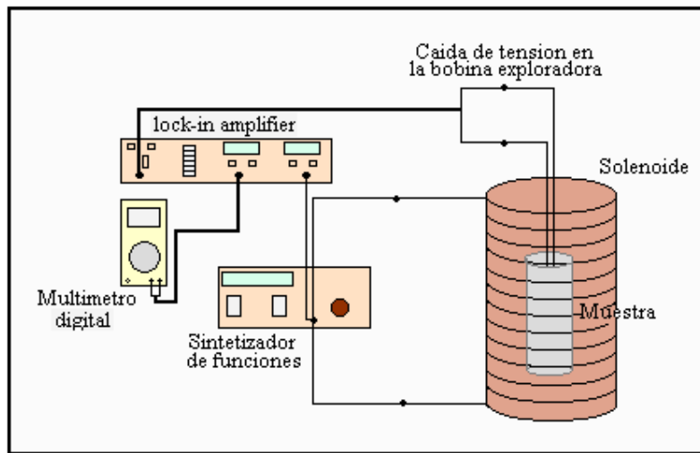
Figura 2: Esquema del dispositivo experimental
