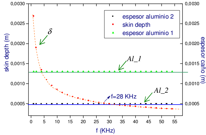
Figura 3: Se grafica el skin depth y el espesor de los caños de aluminio en función de la frecuencia.
