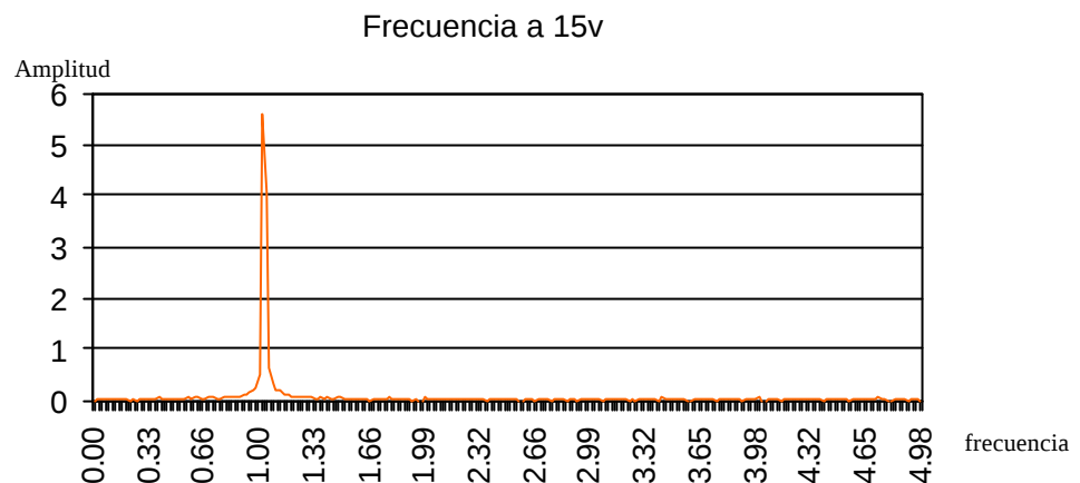
Figura 5: Gráfica de la frecuencia a distancia b(v)=15 vueltas de resorte.
