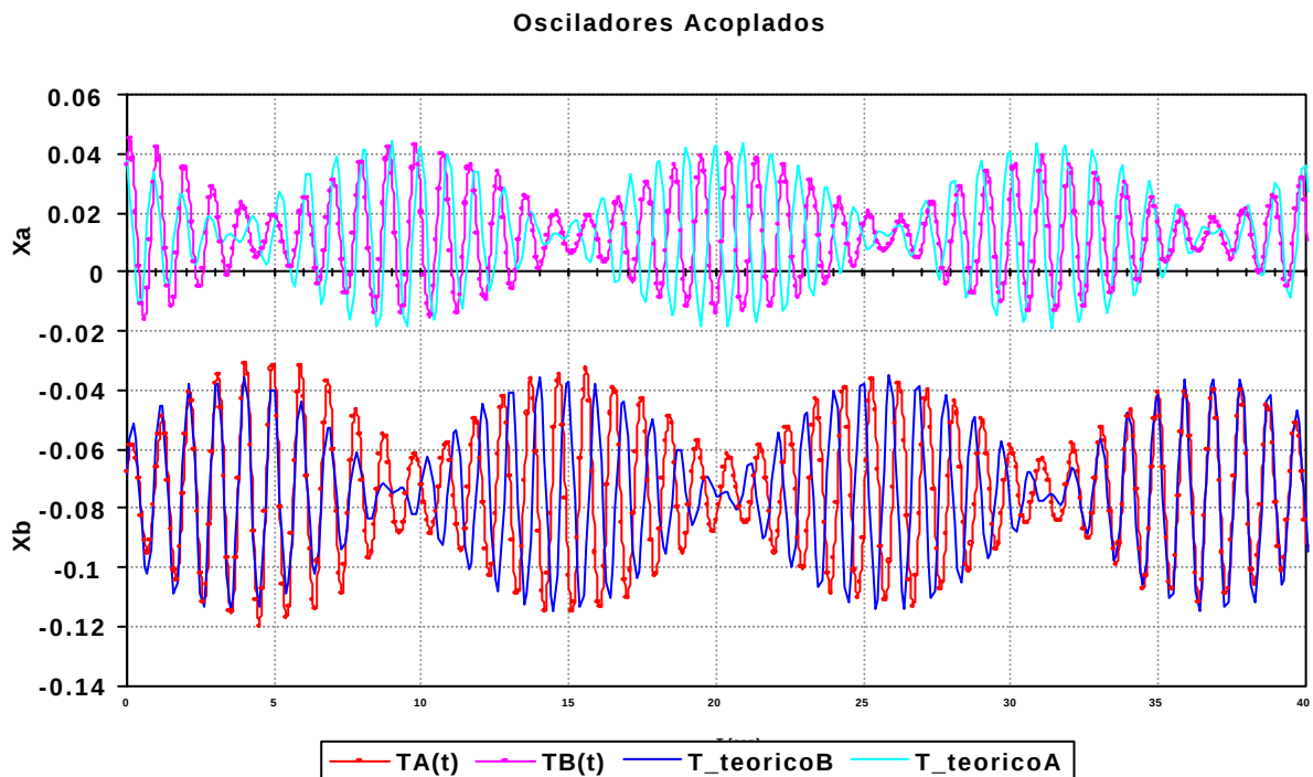
Figura 3: Representación de X_a(t) variando los datos en unidades de x , para obtener una mejor visión y facilitar la comparación.
