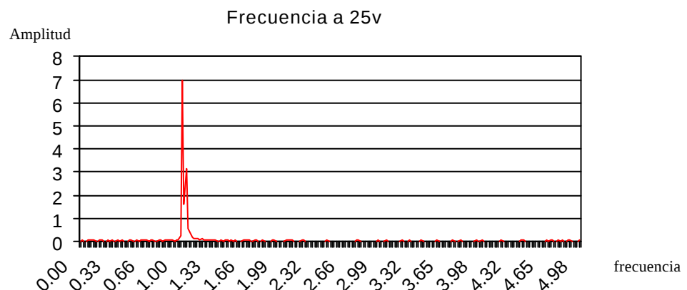
Figura 6: Representación de la frecuencia para el valor de distancia b(v)=25 vueltas de resorte.
