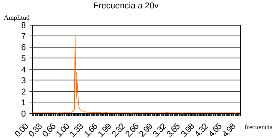
Figura 7: Representación de la frecuencia para el valor de distancia b(v)=20 vueltas de resorte.
