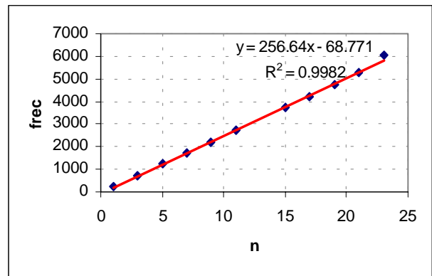
Figura 6 gráfico de la frecuencia en función del orden del modo normal para el tubo chico
