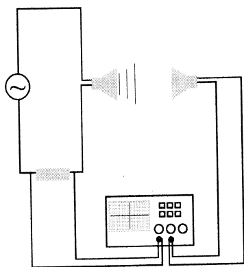
Figura 1: Diagrama del circuito utilizado. El equipo de la parte inferior del dibujo es el osciloscopio, en la parte superior izquierda esta el generador de funciones. El par emisor receptor esta en la parte superior del dibujo
