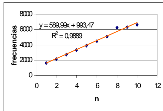
Figura 15: frecuencias de resonancias en función del orden
