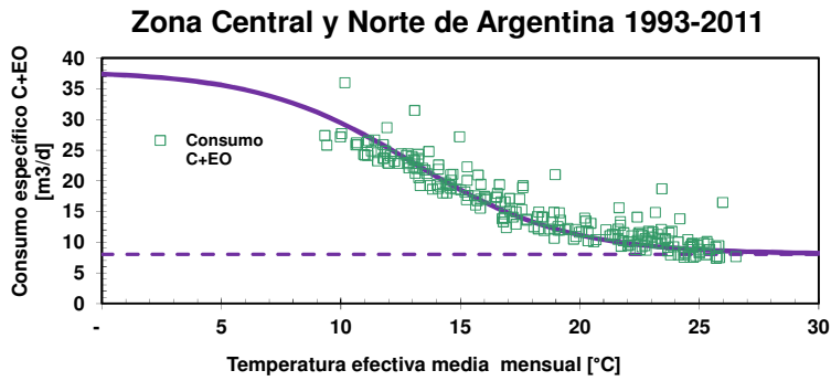
Figura 3. Variación de los consumos específicos comerciales (C) y entes oficiales (EO) como función de la temperatura media mensual. La línea de trazos cortos indica el consumo base su valor es de 8 m 3 /d.
