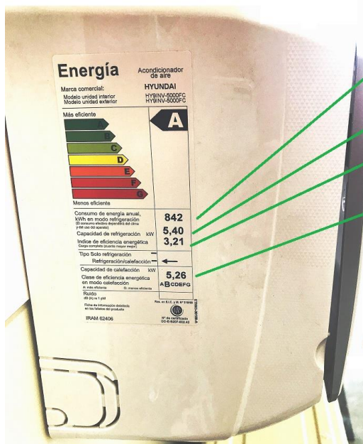
Figura 6. Etiqueta de Eficiencia Energética para acondicionadores de aire según la Norma IRAM 62406 de 2007. El consumo anual corresponde al consumo a máxima potencia (refrigeración) por 50 horas anuales. Abajo se muestra como se relacionan los distintos valores indicados en la etiqueta. La potencia medida a máxima potencia ya sea en calefacción o refrigeración es en general muy cercano al valor del Consumo Eléctrico [kW].
