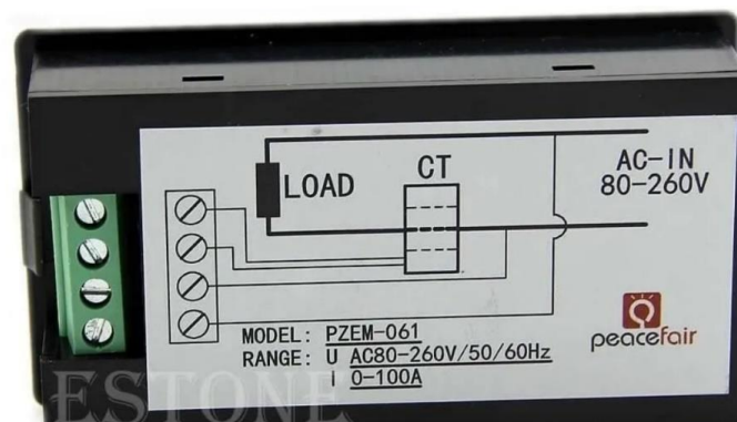
Figura 12: Vista posterior del medidor de consumo. Aquí se indica en modo esquemático en mímico circuito que el de la Figura 1.
