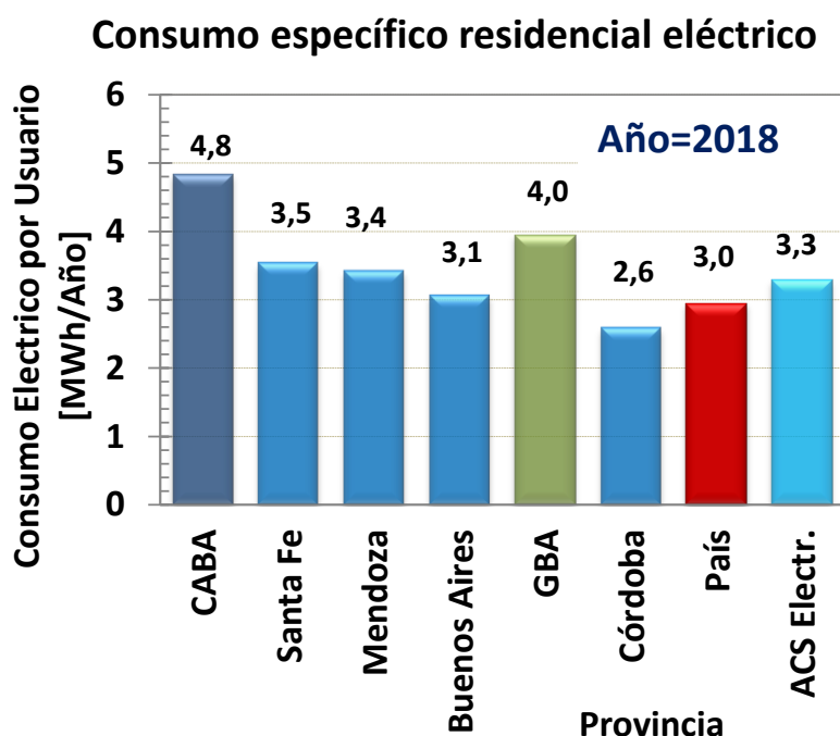
Figura 5. Consumos eléctricos residenciales promedio para las principales regiones de Argentina a partir de los datos de facturación de las distintas distribuidoras. (4) La barra celeste de la derecha, indica el consumo medio de un termotanque eléctrico, de 120 litros, con un consumo medio de unos 180 litros/día. (7) (8) Nótese que en general un termotanque eléctrico es de unos 3,3 MWh/año, equivalente al valor medio del consumo eléctrico nacional.
