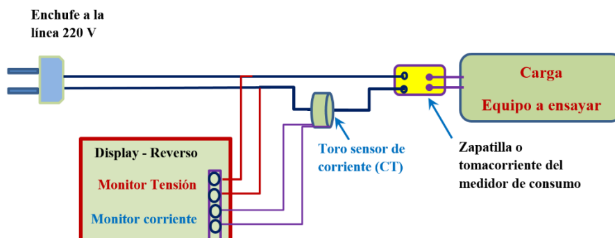
Figura 12: Esquema de conexión del medidor de consumo a un tomacorriente, a donde se conecta el artefacto cuyo consumo se desea medir. Del otro extremo, el medidor de consumo se conecta a la red de 220V.
