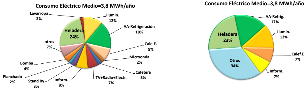
Figura 3. Consumo eléctrico residencial calculado a partir de una muestra de 150 casas de voluntarios de la UNSAM de nivel socioeconómico medio en la región de CABA y GBA. [2] En esta muestra sus habitantes tienen acceso al gas natural. Así el calentamiento de agua se hace principalmente con gas. A la izquierda se muestran la mayoría de los artefactos eléctricos relevados y sus consumos medio. A la derecha, los seleccionamos los principales consumos eléctricos de la misma muestra.
