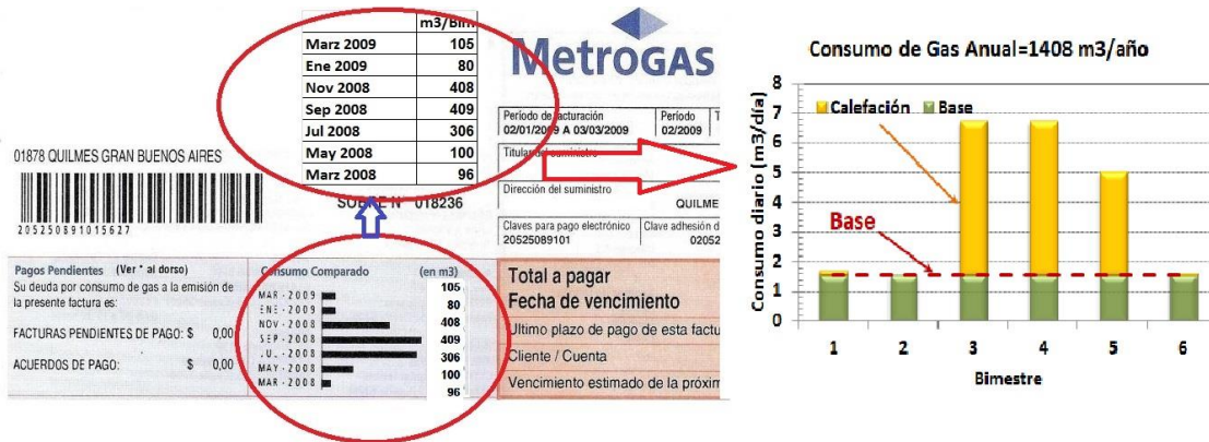
Figura 7. Consumo de gas: a partir de las facturas de gas, (Izquierda) puede obtenerse el consumo por bimestres de los 6 o 7 últimos bimestres. Dividiendo por el número medio de días por bimestres (60,8 días), se puede obtenerse el consumo medio diario por bimestre. Suponiendo que en los bimestres estivales no se usa la calefacción, promediando estos consumos estivales se obtiene el consumo medio base, asociado al uso de cocción u calentamiento de agua. El consumo por encima de este valor en los meses invernales, nos dan una idea del consumo de calefacción.
